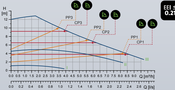
MAGNA1 25-120 (N)
